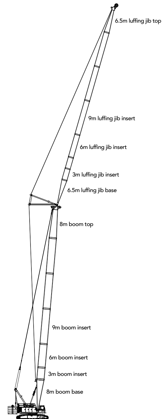
LJ Configuration (22m~52m)+(22m~52m)
